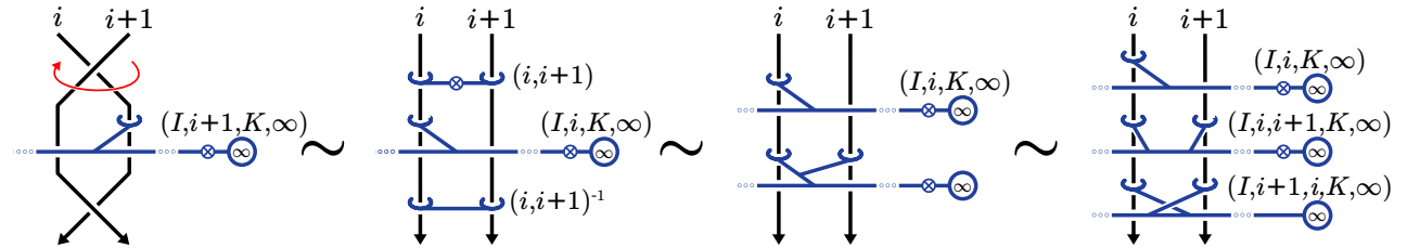
FIGURE 15. Computation of (d).
